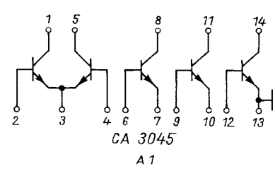
Bild 3: Anschlußbelegungen zu Tabelle 3
