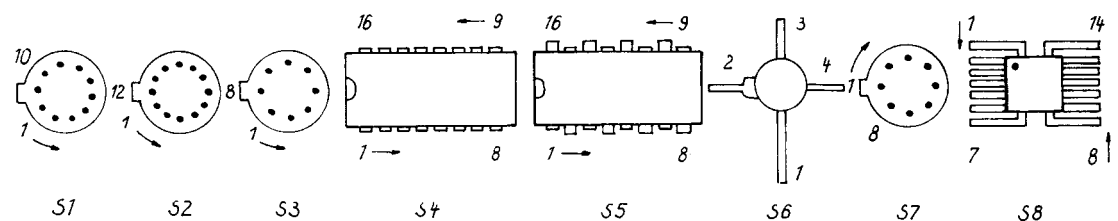
Bild 4: Sockelbilder (S1, 2, 3, 7 von unten)
