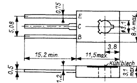
Bild 5: Maßbild für die identischen Gehäuseformen TO-126 und SOT-32. Oben ist die Draufsicht gezeigt, d. h., das galvanisch mit dem Kollektor verbundene, in das Plastikgehäuse eingelassene Kühlblech befindet sich unten.
