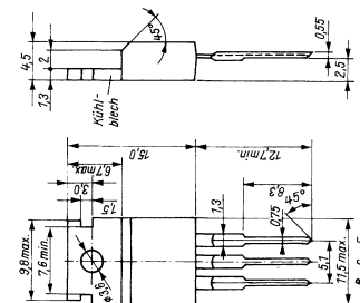
Bild 6: Abmessungen und Anschlußbelegung des Gehäuses TO-220-A. Die Kühlfahne führt Kollektorpotential. Links die Draufsicht. Dieses Gehäuse ist dem Typ SOT-78 sehr ähnlich.
