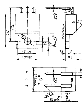
Bild 7: Gehäuse TO-220-B. Auch hier sind zwecks optimaler Wärmeabfuhr Kollektor und Kühlfahne leitend verbunden.
